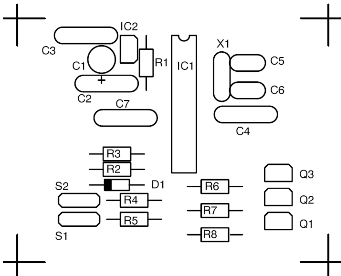
Implantation des composants
