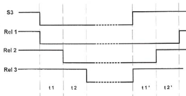
Figure 1: Diagramme de commutation des relais
