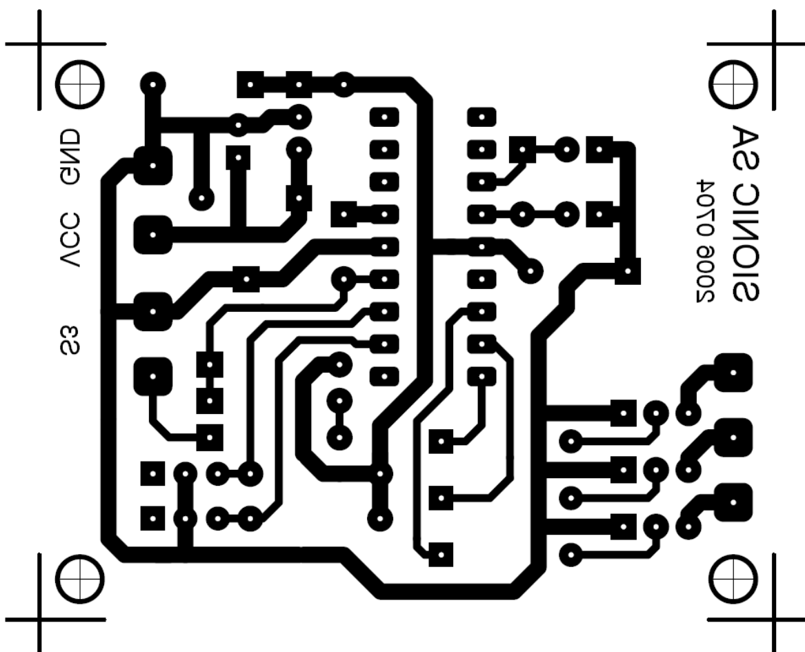
Circuit imprimé vu côté circuit
