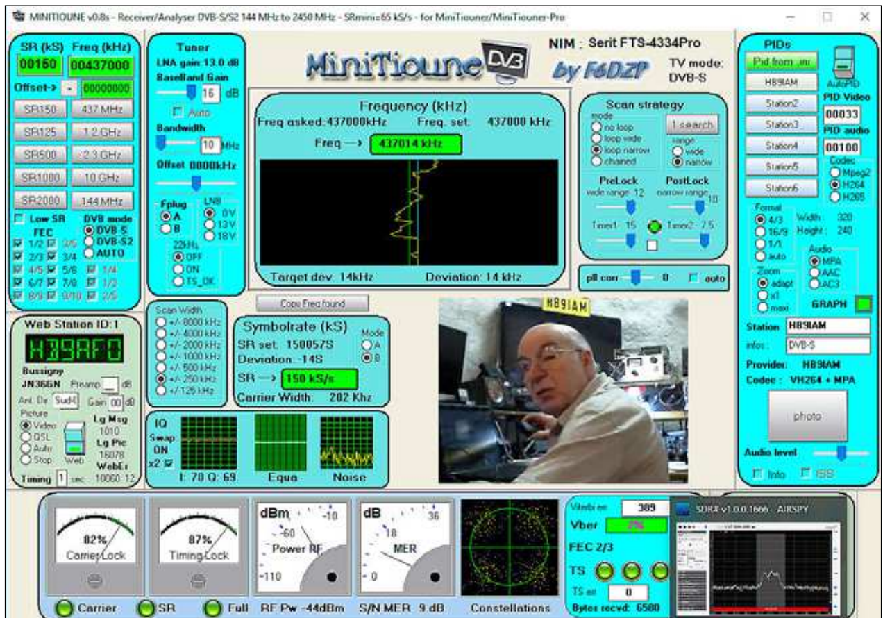
Fig. 3 - Minitioune lors de la réception de Pierre Binggeli HB9IAM (membre d'honneur de l'USKA) via le Mont Blanc
